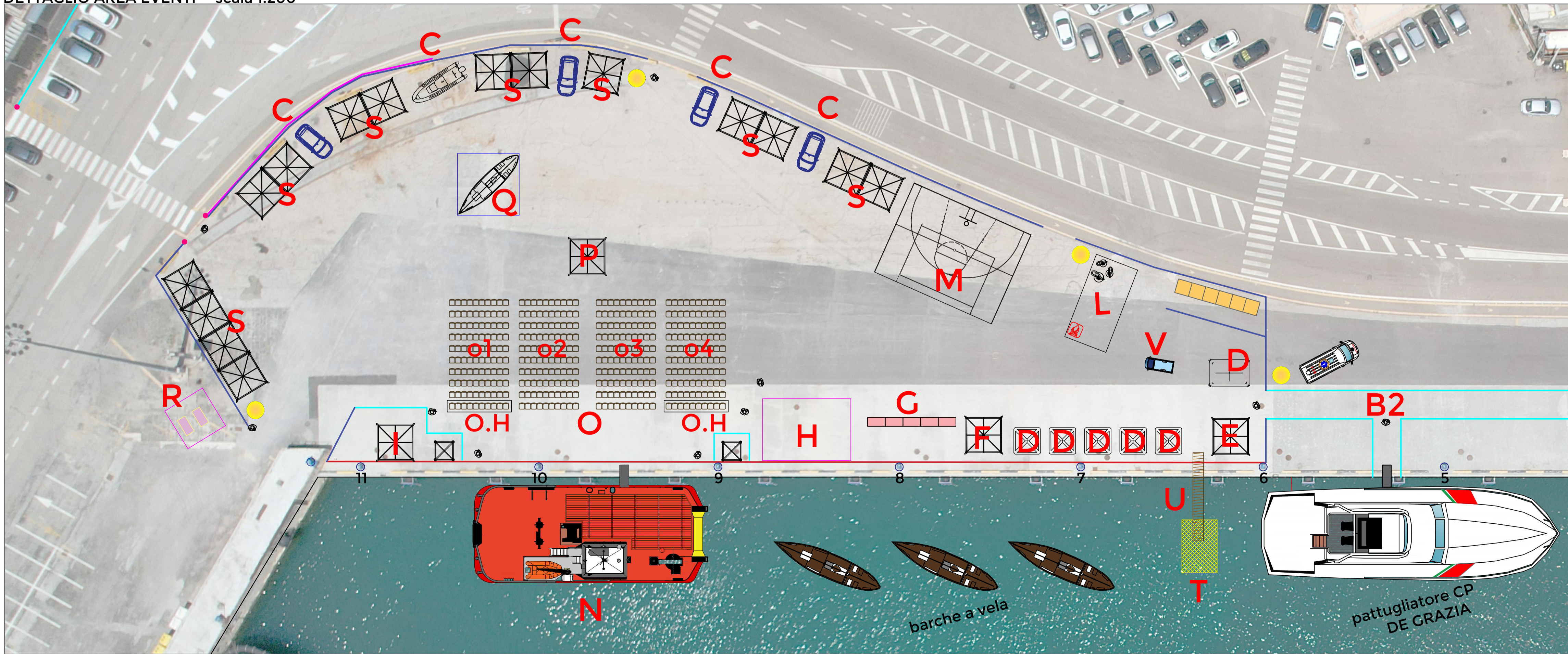
DETTAGLIO AREA EVENTI - scala 1:200
